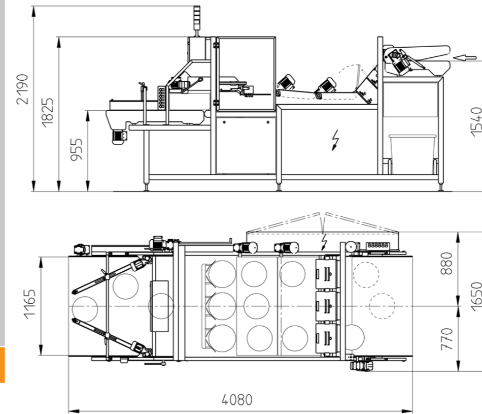
Propuesta de layout no vinculante.
